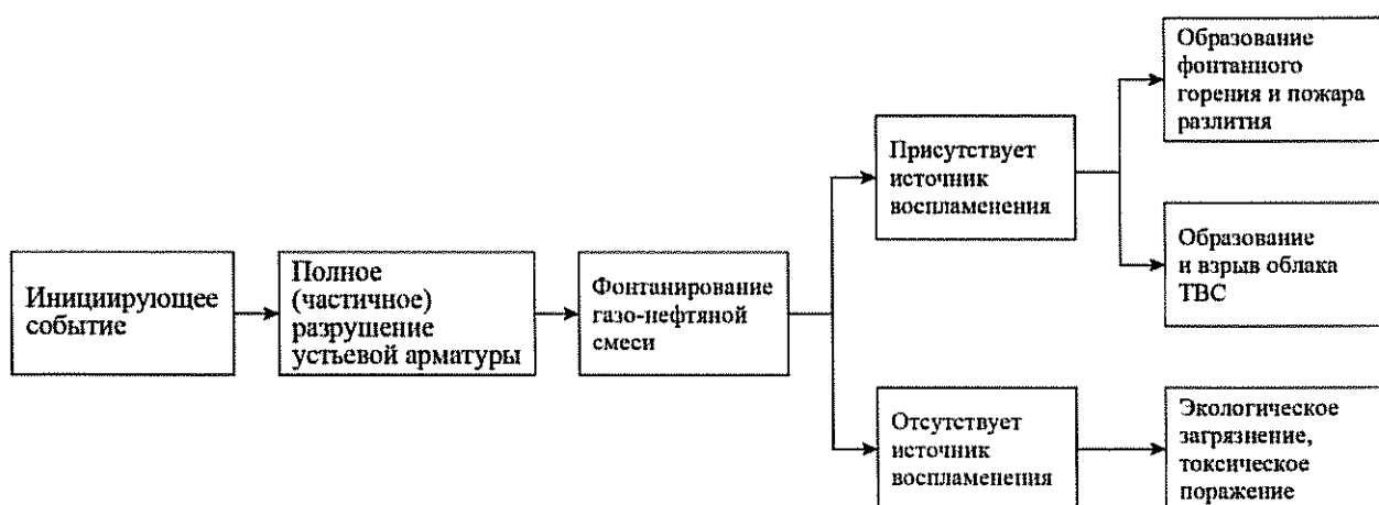
Рис. 10. «Дерево событий» при разрушении устьевой арматуры нефтяных фонтанирующих скважин (сценарий A_{10} )
