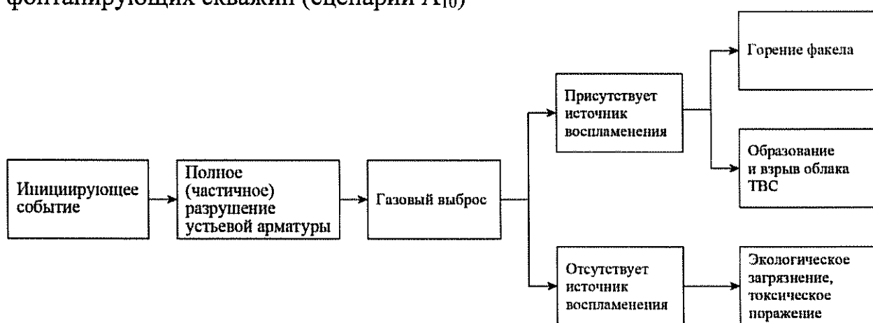
Рис. 11. «Дерево событий» при разрушении устьевой арматуры нефтяных фонтанирующих скважин (сценарий A_{10} )
