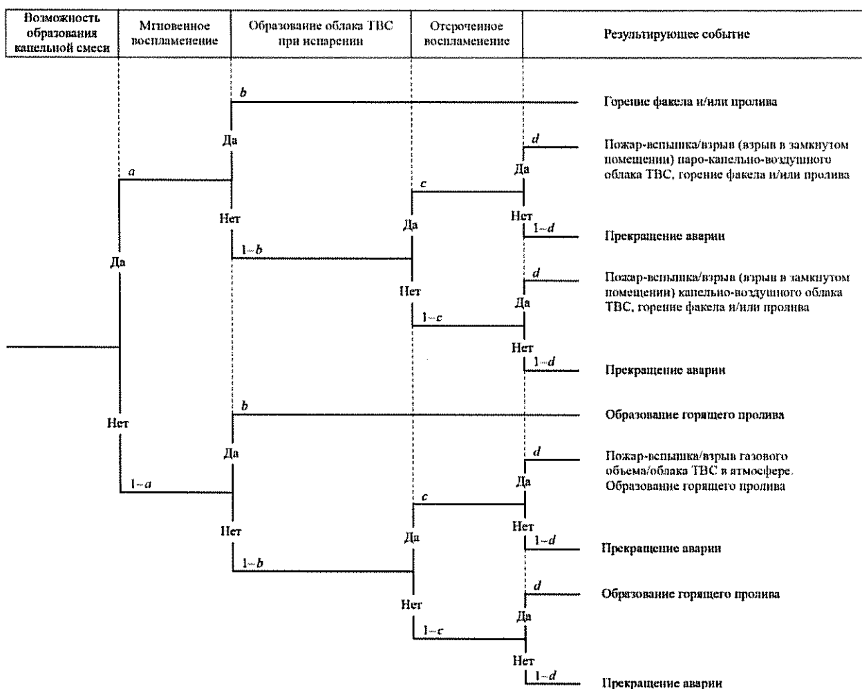
Рис. 9. «Дерево событий» при аварии в насосных (сценарий А 9 )
